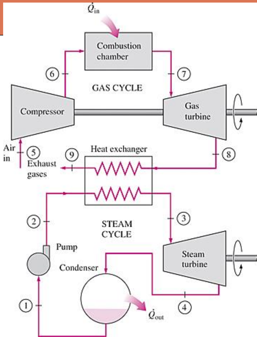
Birleşik gaz-buhar güç santrali.
